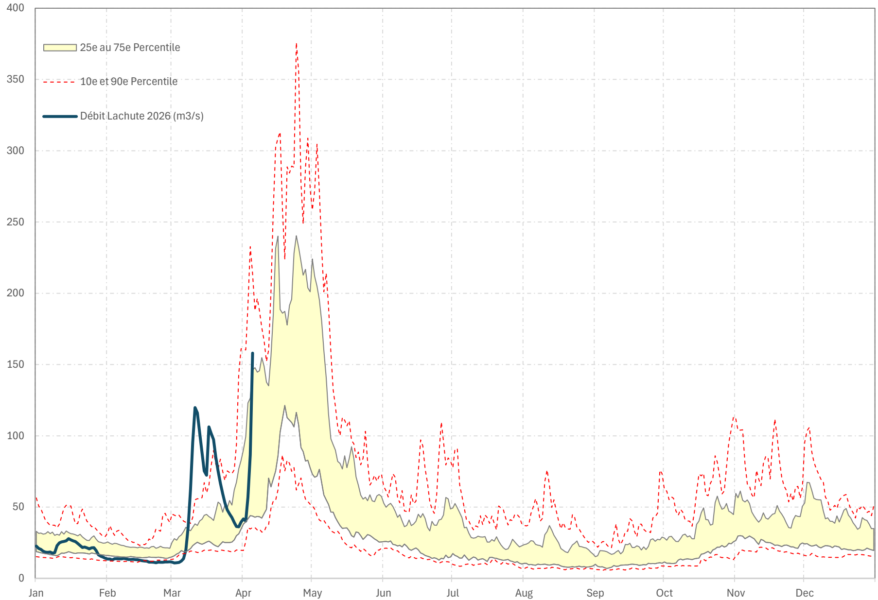
Débit Rivière du Nord à Lachute [Moyenne Journalière]
